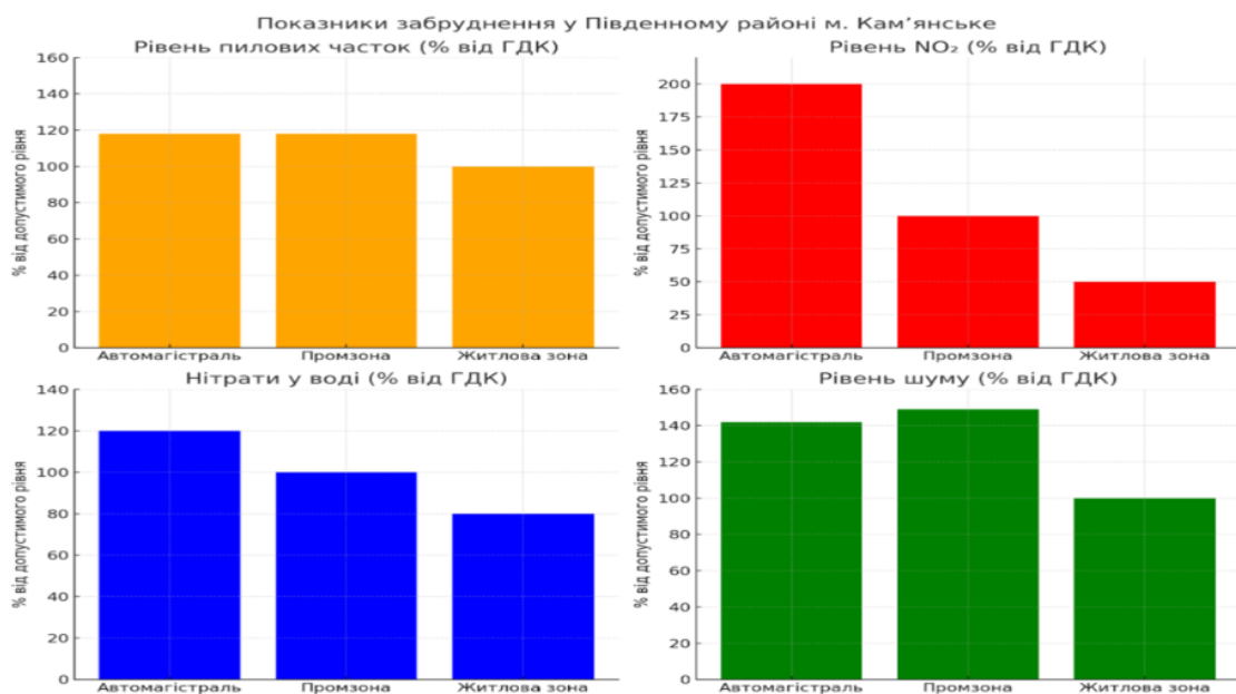
Рис. 1. Показники забруднення у Південному районі м. Кам'янське (у відсотках до ГДК).
