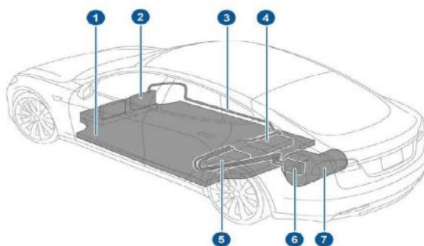
Рис. 4. Високовольтні компоненти електромобіля.
