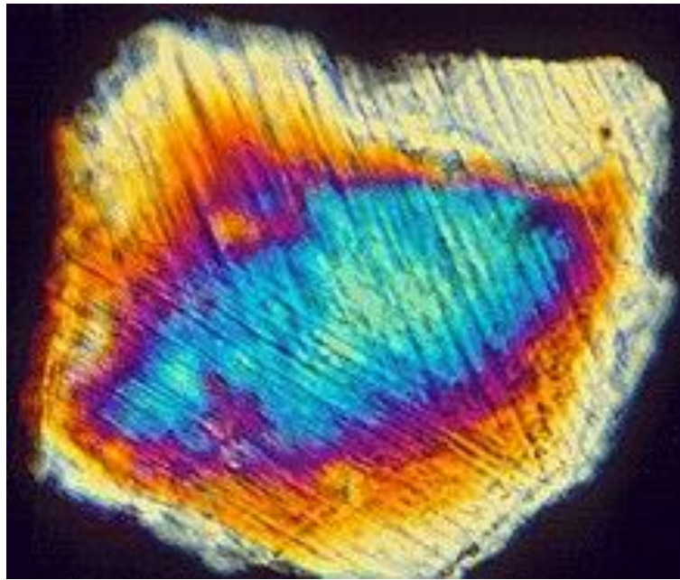
Рис. 6. Шоковий кварц
